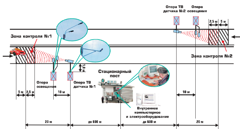
Схема размещения стационарного АПК «Поток» в на типовом стационарном посту
